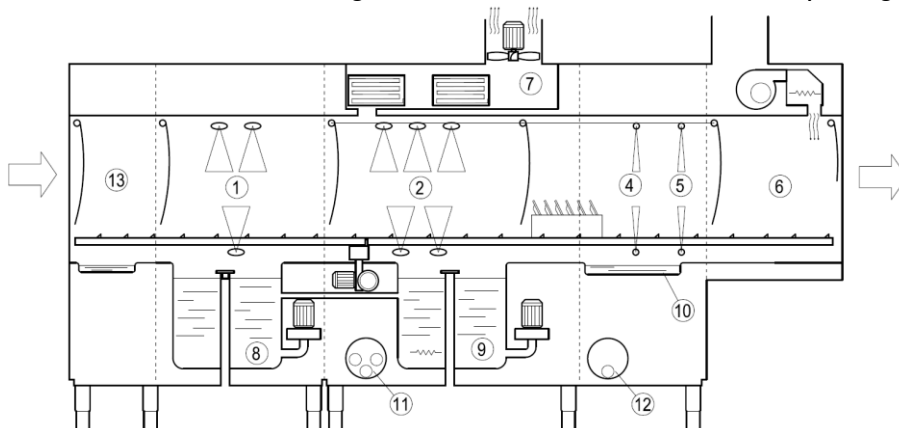
Schematische Darstellung der Maschine mit Zwei-Phasen-Spülung
