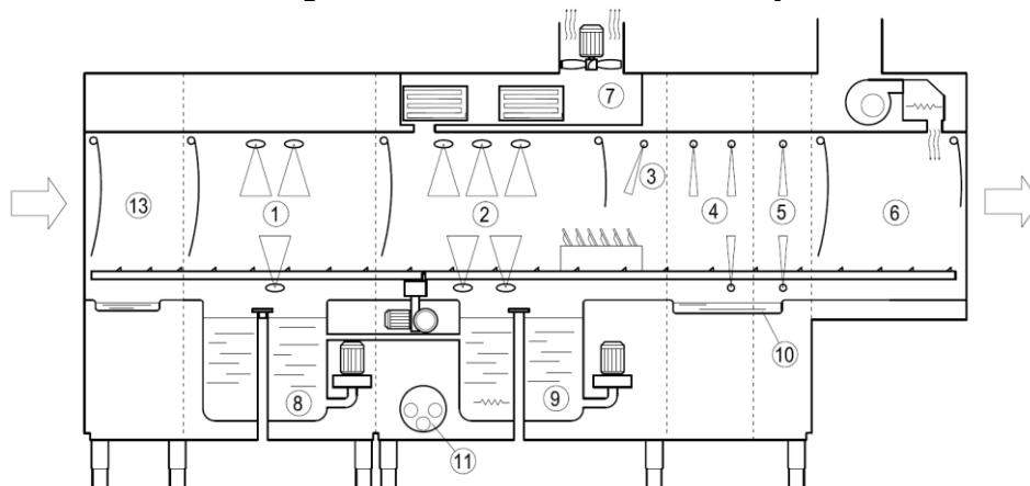
Diagram over maskinen med multiskyl
