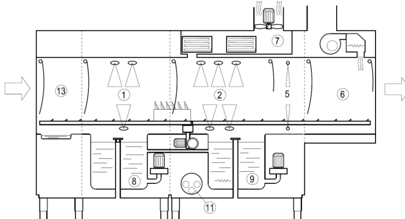
Διάγραμμα του μηχανήματος με μονό ξέπλυμα
